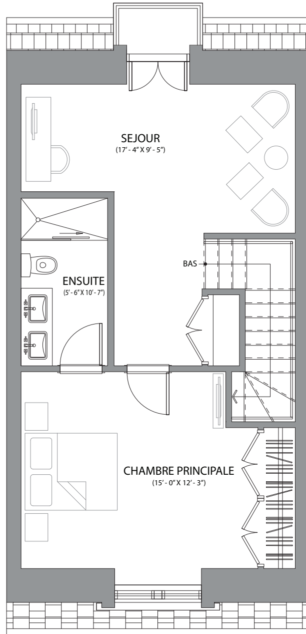
Plan du troisième étage
