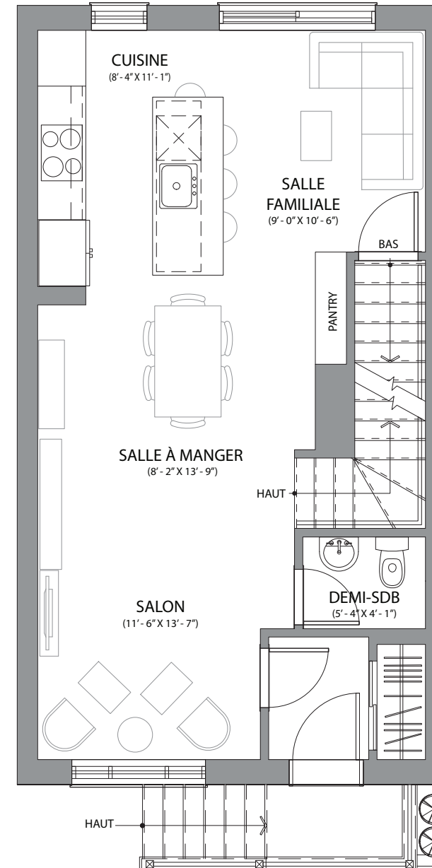
Plan du rez-de-chaussée
